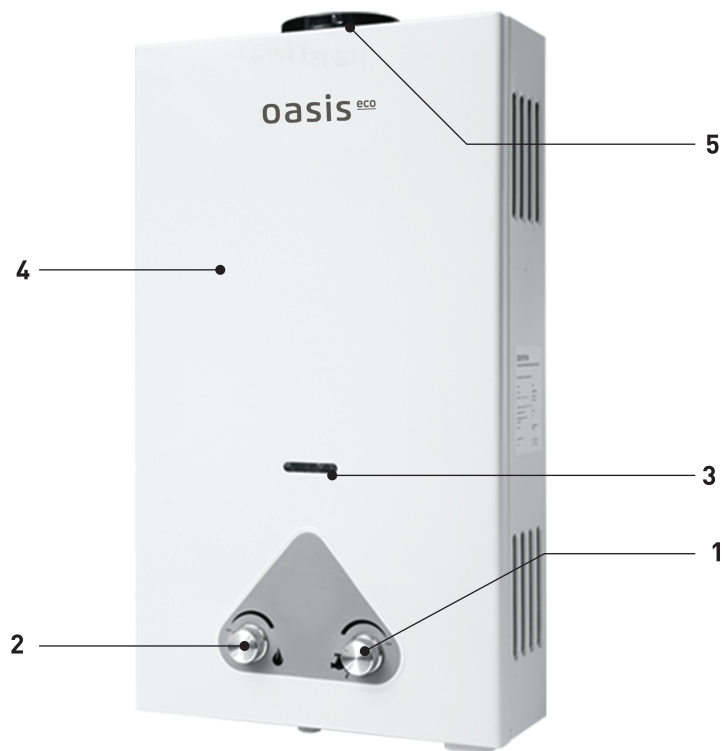
Рис. 1. Аппарат водонагревательный проточный газовый бытовой Oasis Eco 1 - ручка водяного регулятора; 2 - ручка газового регулятора; 3 - окно смотровое; 4 - облицовка ; 5 - патрубок дымоотвода.
